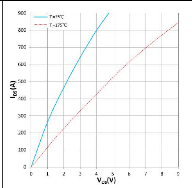
Figure 6. I_{DS} vs V_{DS} V_{GS} = 15\text{V} , T_j parameter
