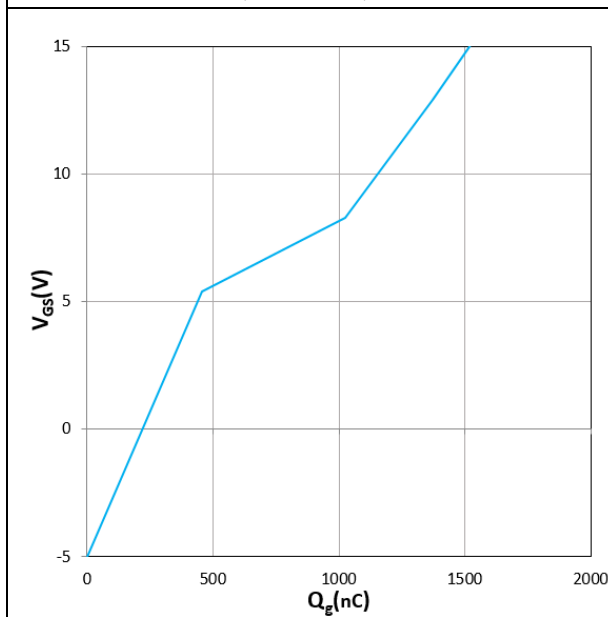
Figure 11. V_{GS} vs Q_g T_j = 25^\circ C , V_{DS} = 1000V , I_D = 450A
