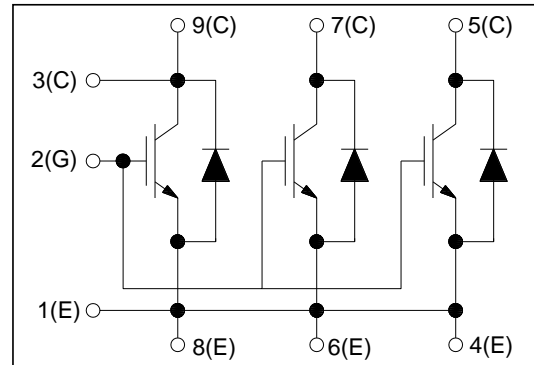
图 1. 电路结构
