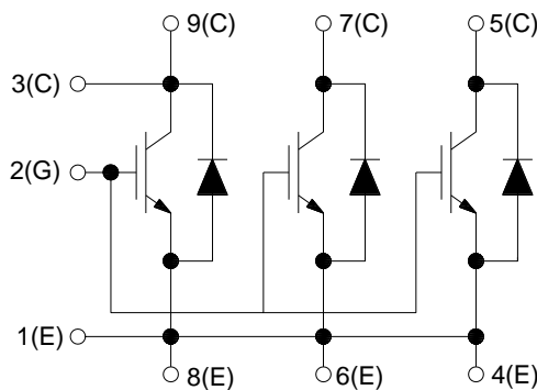
图 1. 电路结构
