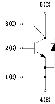
图 1. 电路结构
