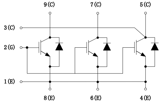
图 1. 电路结构 Fig. 1 Circuit configuration
